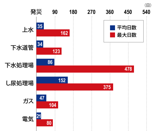
東日本大震災自治体におけるライフライン別の 仮復旧までの日数(回答29自治体) (日本トイレ研究所)
